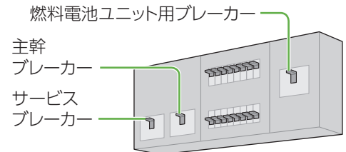
家庭用燃料電池対応分電盤
